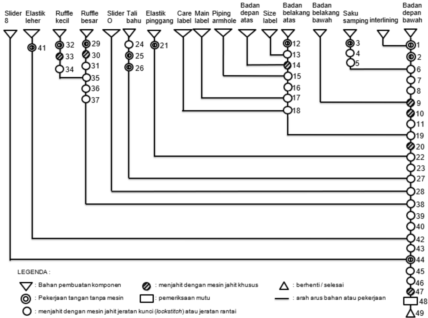
Lampiran 2. Operation Process Chart (OPC) untuk H&M Apple Jumpsuit White Light AOP
