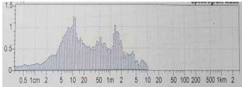
Gambar Spectrogram Sliver Carding Sebelum Perbaikan Menggunakan Alat Uster Tester 5
