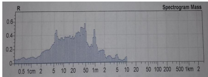
Gambar Spectrogram Sliver Carding Setelah Perbaikan Menggunakan Alat Uster Tester 5
