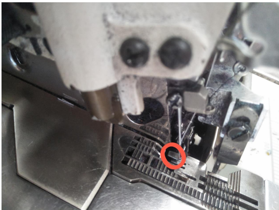
Lampiran 5. Lidah pada Plat Mesin Obras Benang 5
