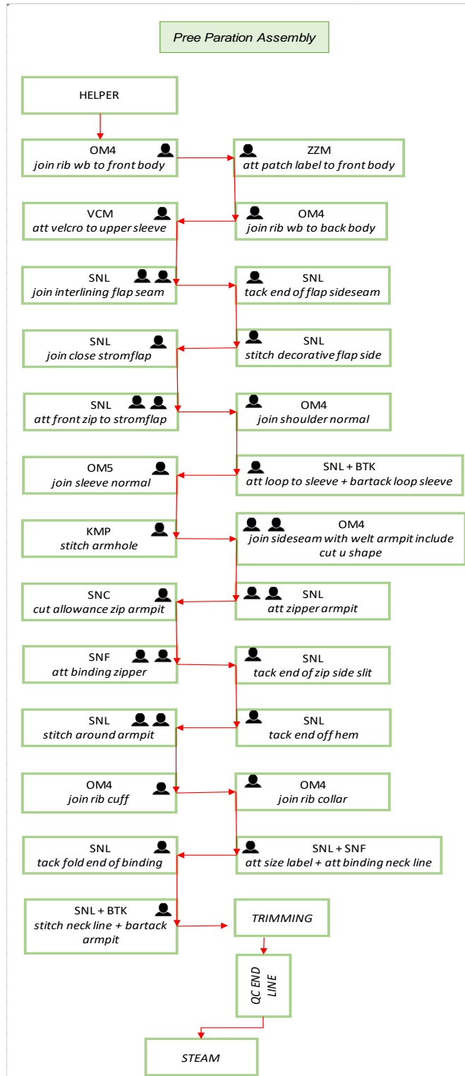
Lampiran 1 Layot Proses Pembuatan Jaket Style PSIM
